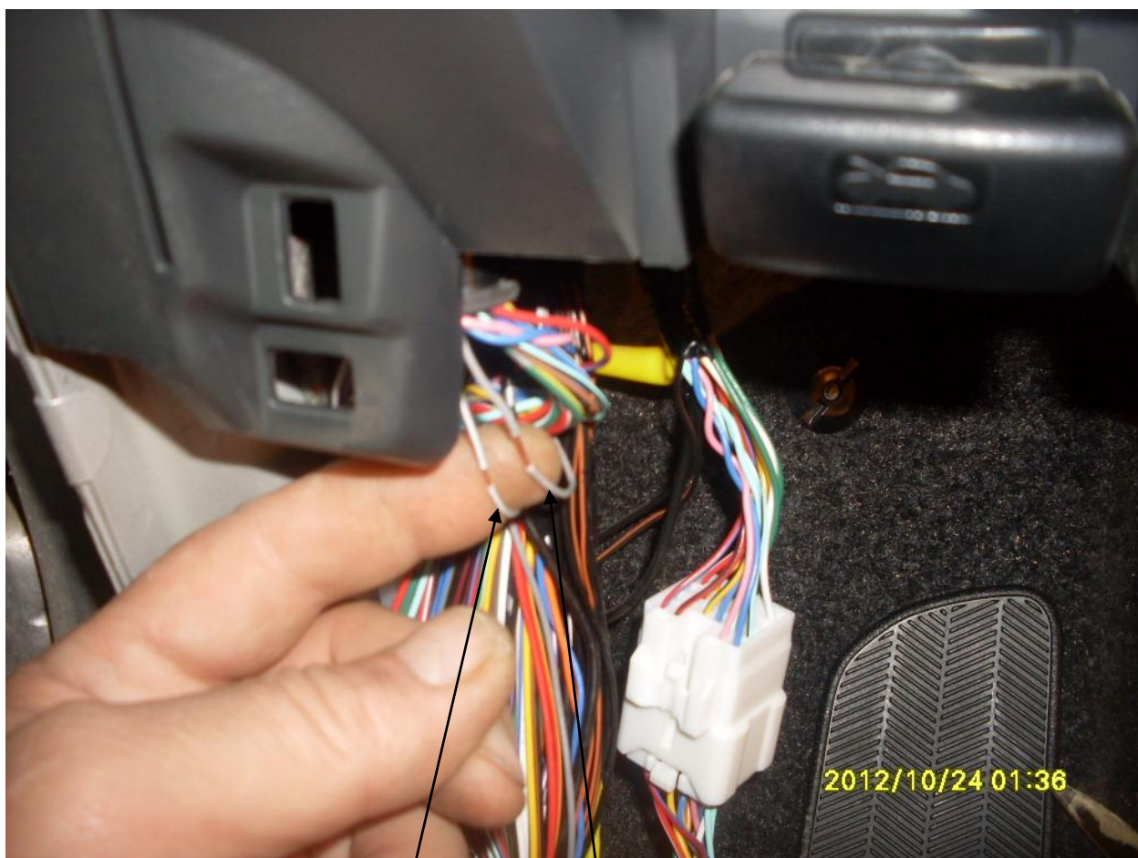
Жгут из двери водителя Ц.3 серо-белый закр. серый откр. минусовое управление.
